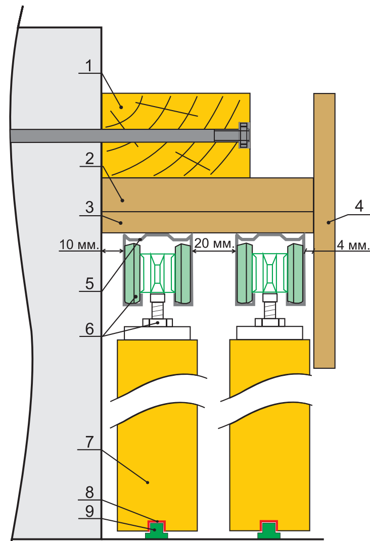
Схема монтажа №1
