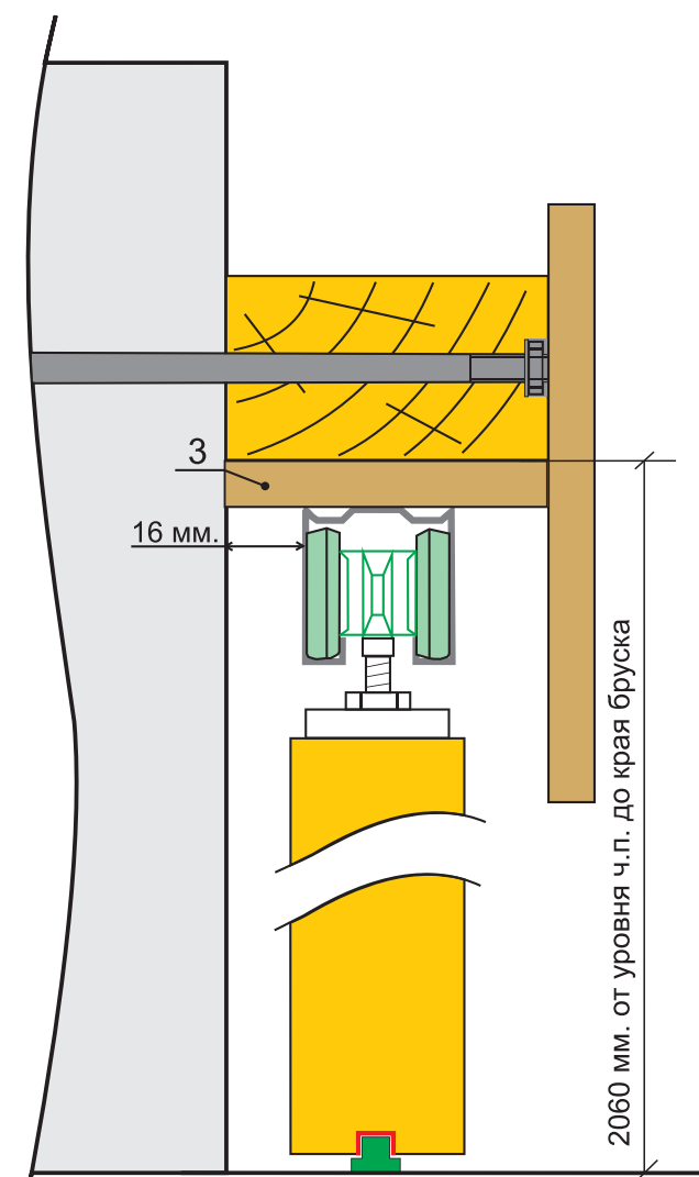
Схема монтажа №2
